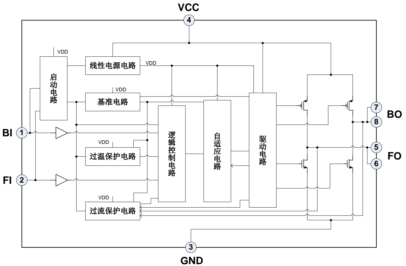
图 2. 主要模块框图
