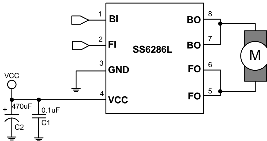
图 4. 应用原理图
