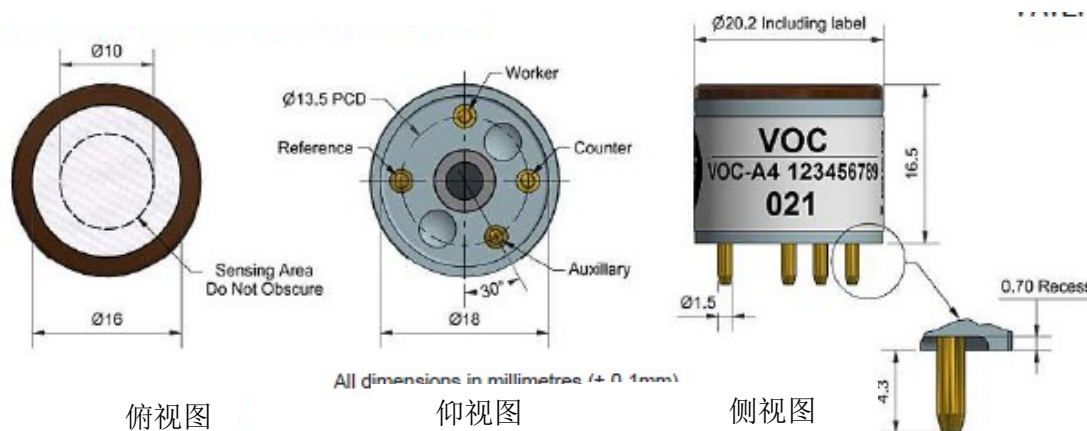
图1 VOC-A4示意图
